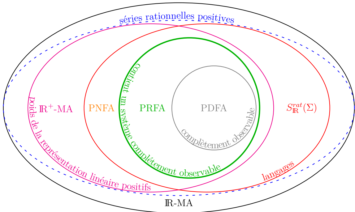
FIGURE 7.1 – Hiérarchie entres les classes d'automates. Dans ce chapitre, nous nous intéressons à la classe d'automate en vert épais.
