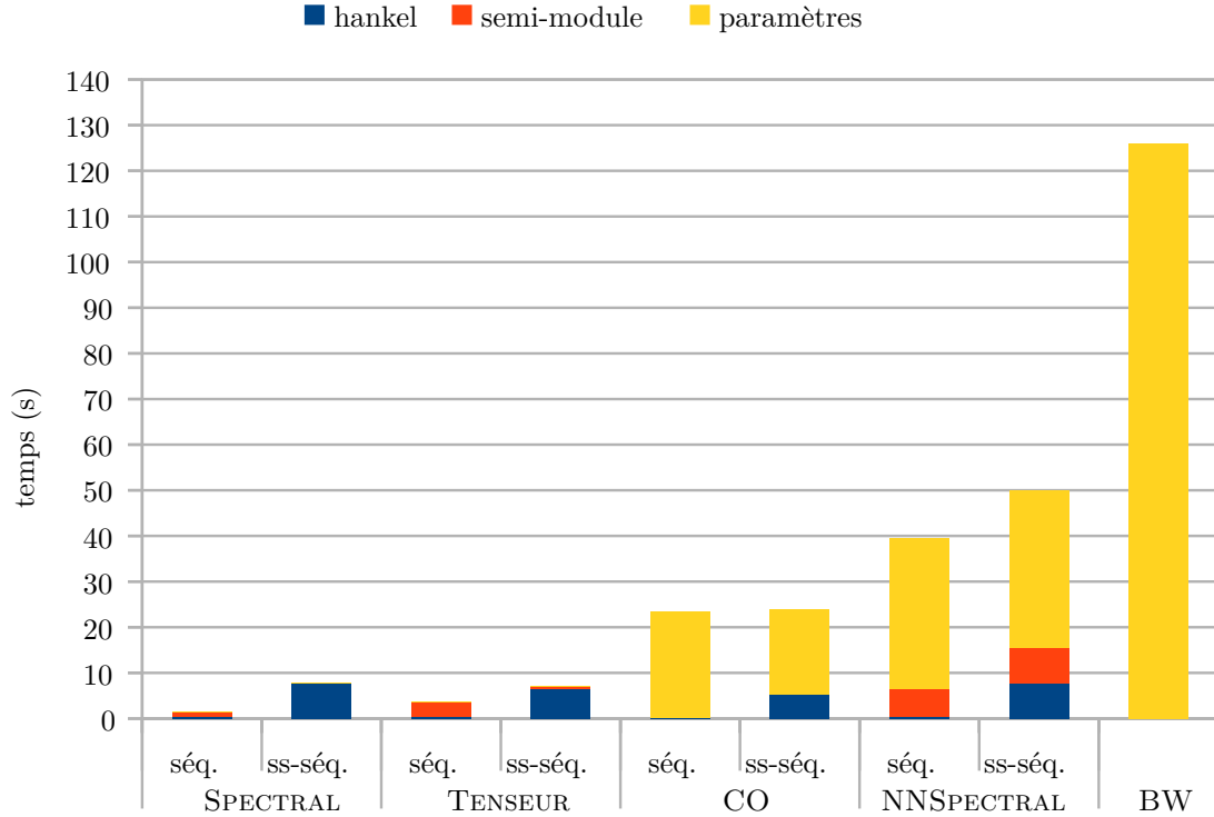
FIGURE 5.2 – Temps d’exécution moyen par algorithme sur douze problèmes de PAutomatC.
