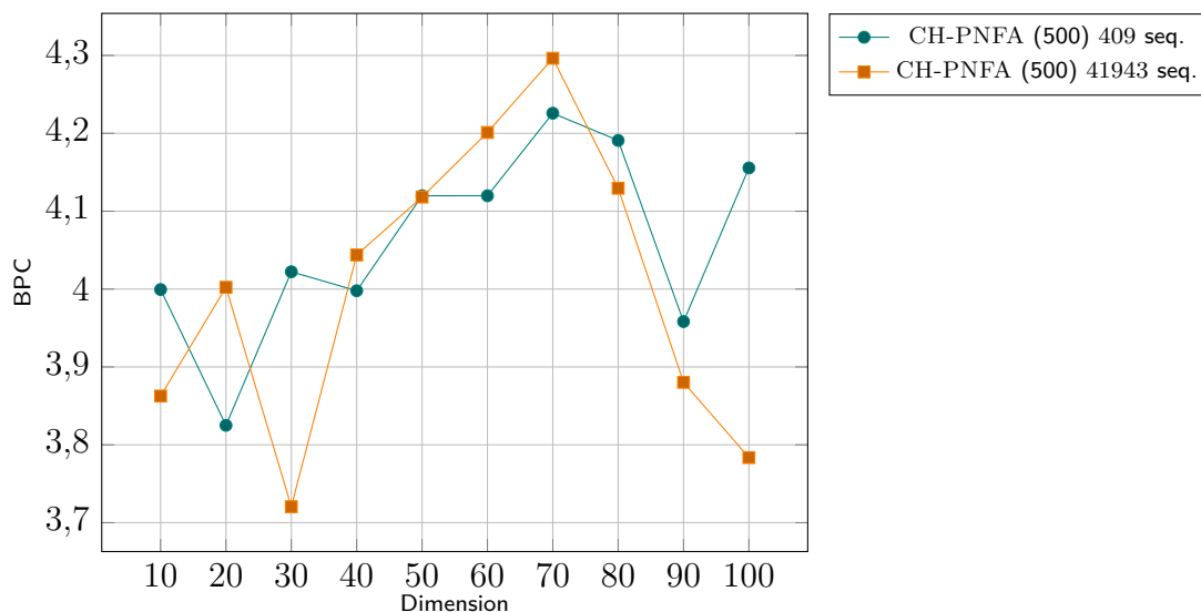
FIGURE 6.3 – Performances de CH-PNFA et NNSPECTRAL pour le BPC sur 41943 séquences extraites de Wikipédia en fonction de la dimension.
