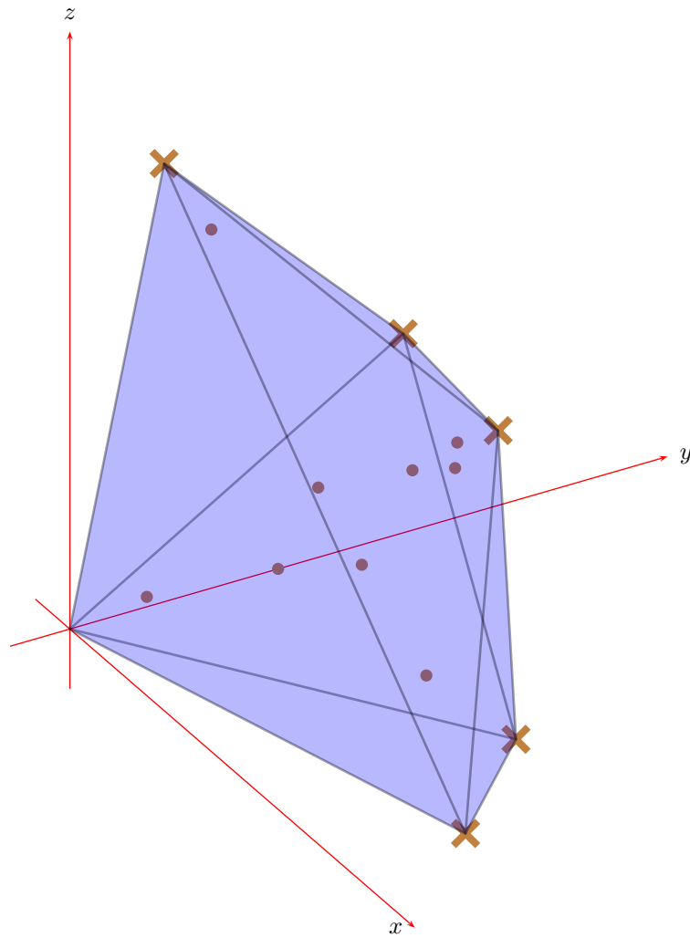
FIGURE 7.3 – Enveloppe convexe d'un ensemble de vecteurs et de l'origine. Les séries \{up|u \in \mathcal{P}\} , formant les lignes de H_{\mathcal{B}} , sont représentées sous forme de vecteurs définis sur \mathcal{S} en marrons. Les croix marrons sont les séries \{up|u \in \mathcal{R}\} . Elles supportent l'enveloppe convexe contenant les autres séries (et l'origine), représentées par les points marrons.
